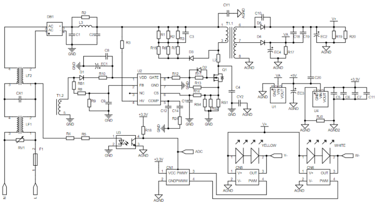
原理图
