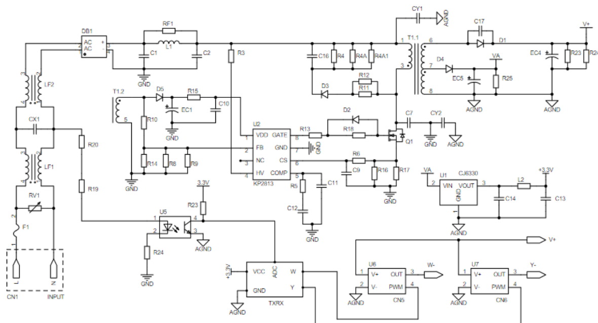
原理图
