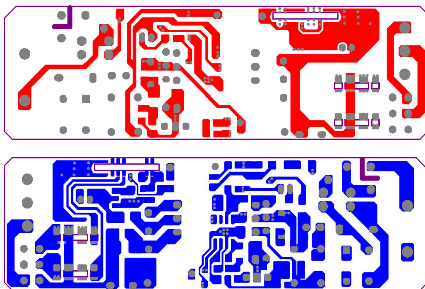
PCB 板图
