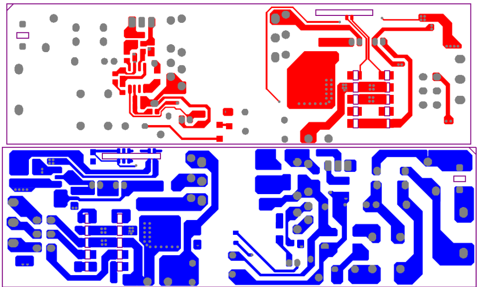
PCB 板图
