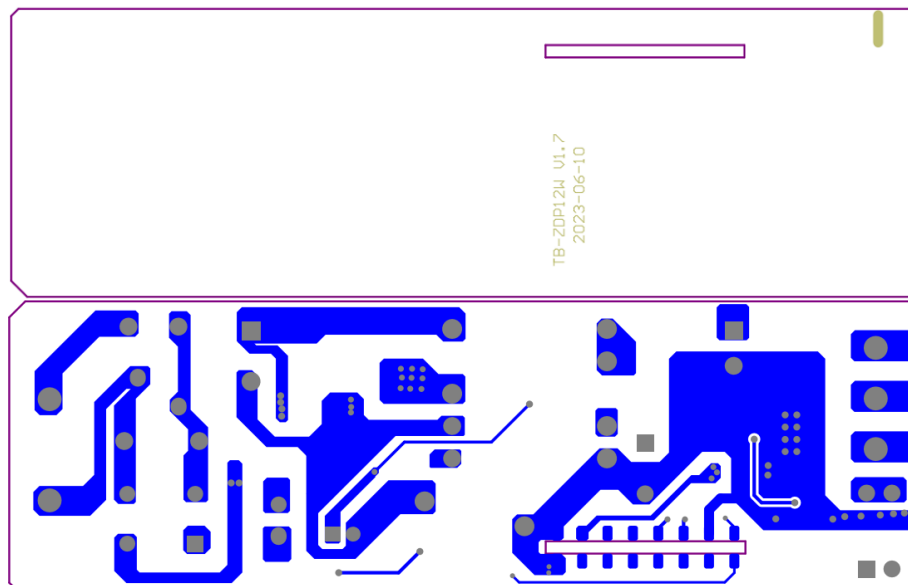
底层 PCB 图
