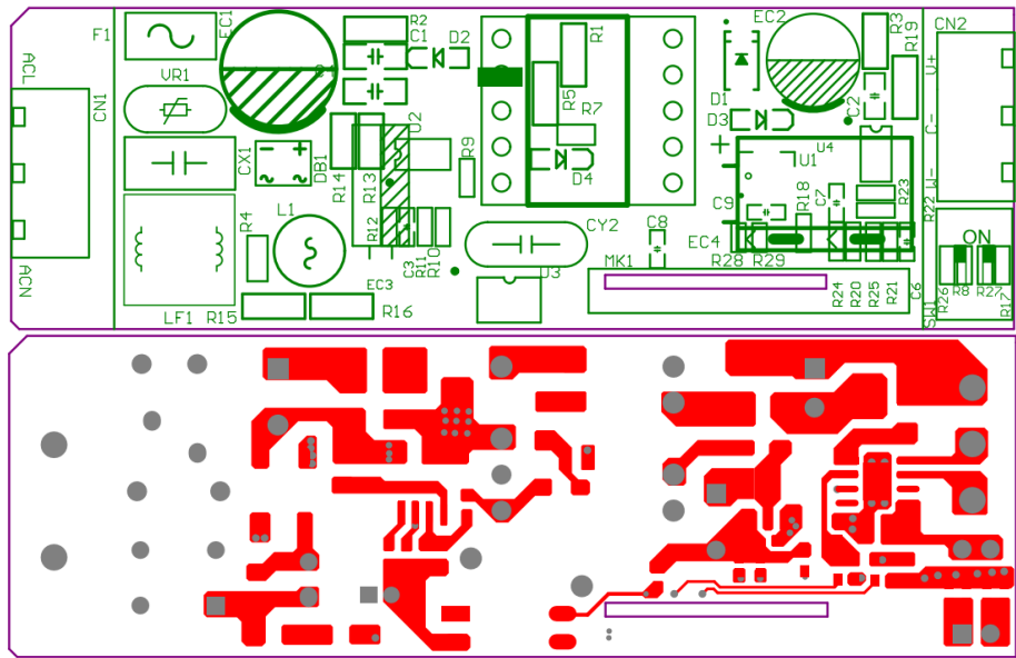
顶层 PCB 图
