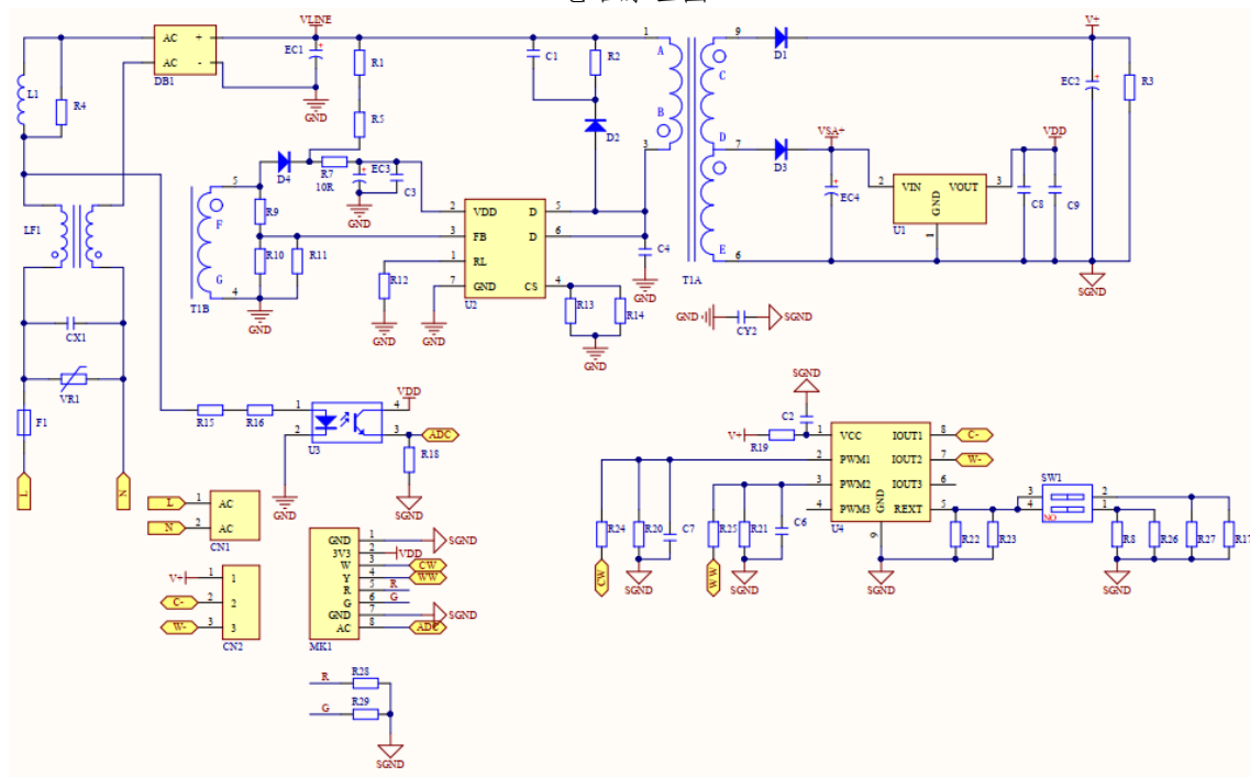
电路原理图
