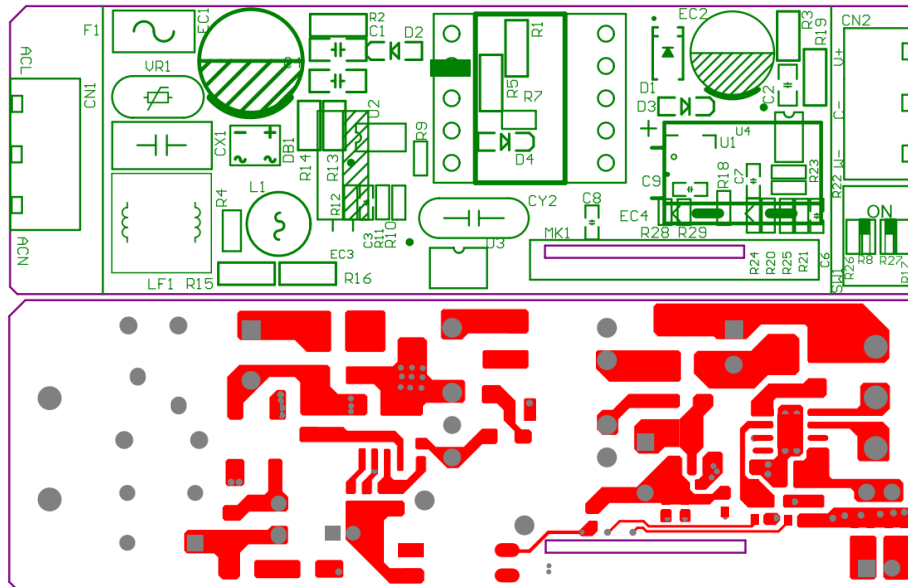
顶层 PCB 图
