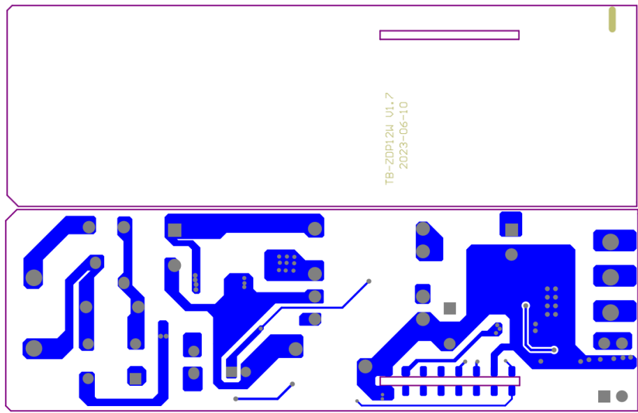
底层 PCB 图
